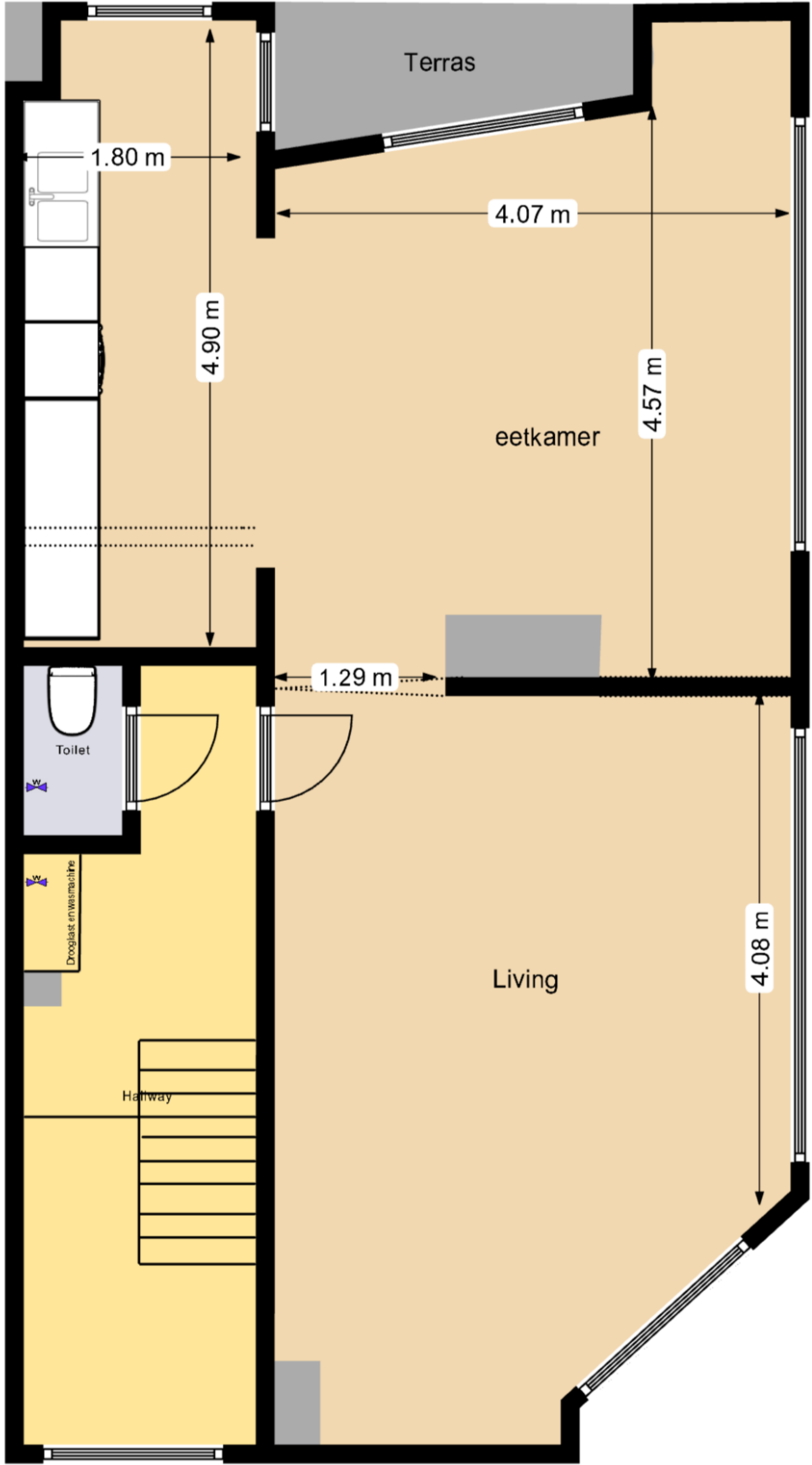
Eerste verdiep
